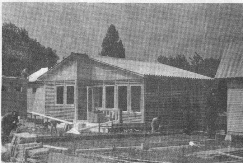
4. sz. fénykép: Csaknem kész faházunk a Budapesti Nemzetközi Vásáron (Bognár Antal felvétele)
