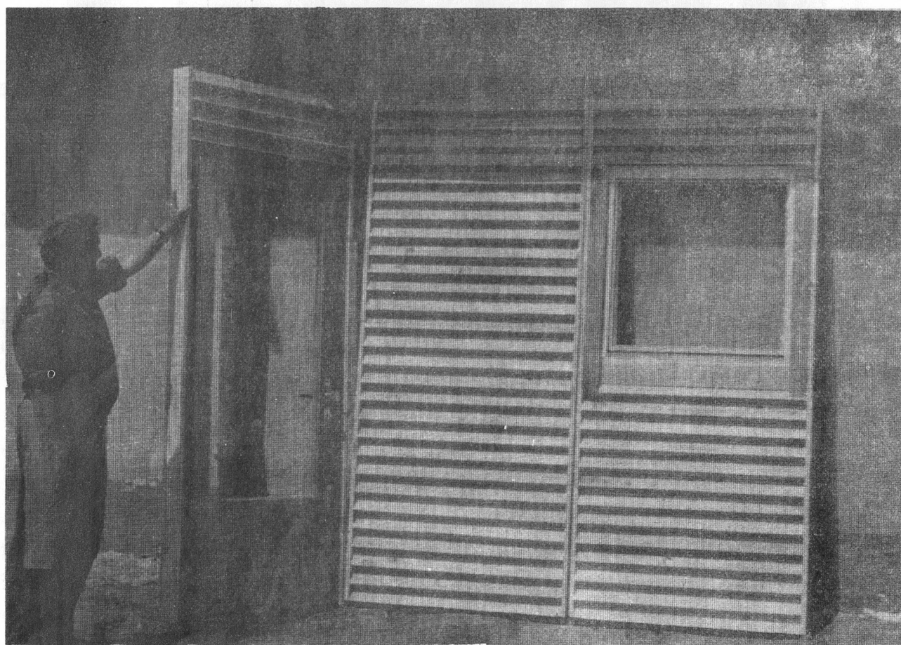
2.-3. sz. fénykép: A faház elemeinek összerakása építés közben (Bognár Antal felvétele)
